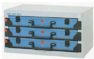
Réf./ref. D 973883 DIMA TURM 388/3 Vide/ledig 555x350x290 mm Pour/voor: 3 x DIMA 88/2
