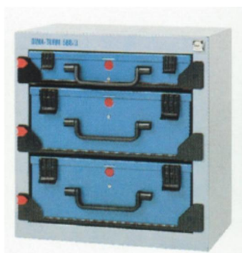
Réf./ref. D 9735883 DIMA TURM 577/3 Vide/ledig 416x256x434 mm Pour/voor: 1 x DIMA 88/1 2 x DIMA 88/3
